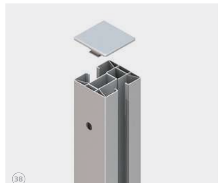
Klemmpfosten
