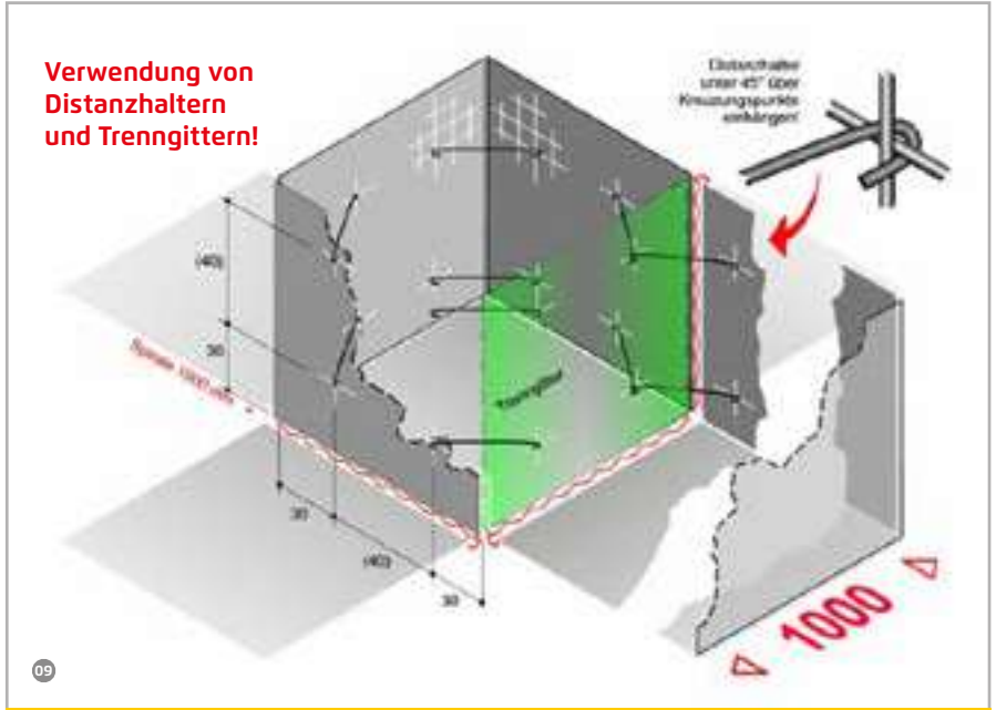
Schemazeichnung 1 – Korbtiefe 1000 mm / Korbbreite max. 1000 mm!
