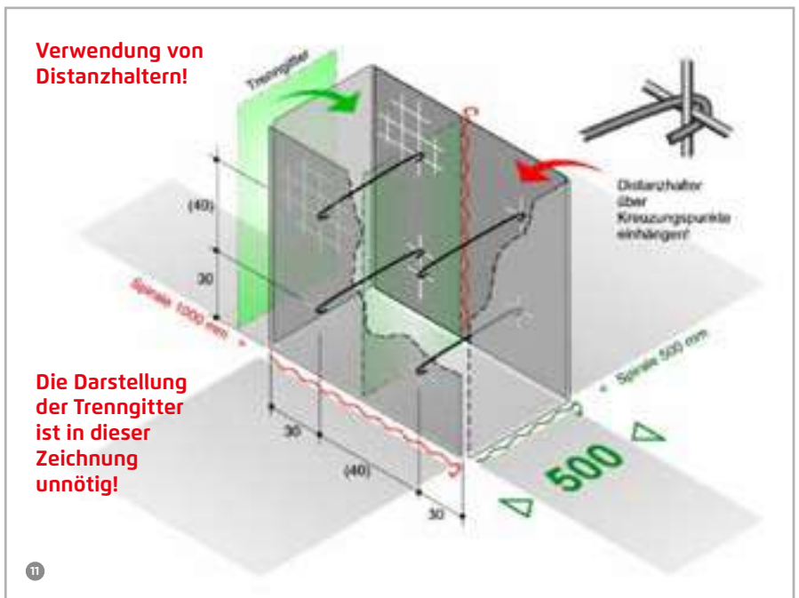
Schemazeichnung 2 – Korbtiefe 500 mm!
